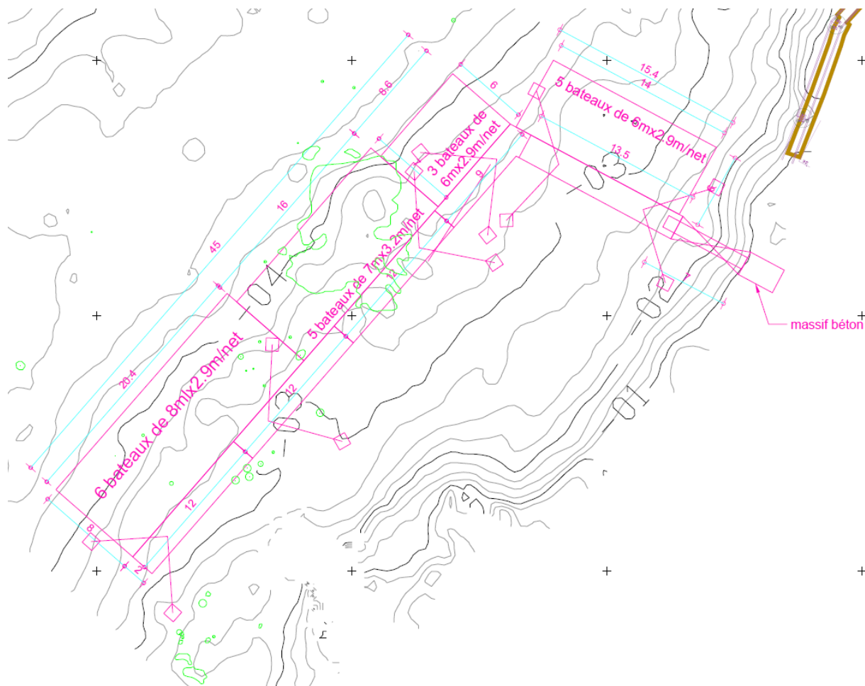
Vue en plan du ponton SCP (TP SPADA, 2023)
